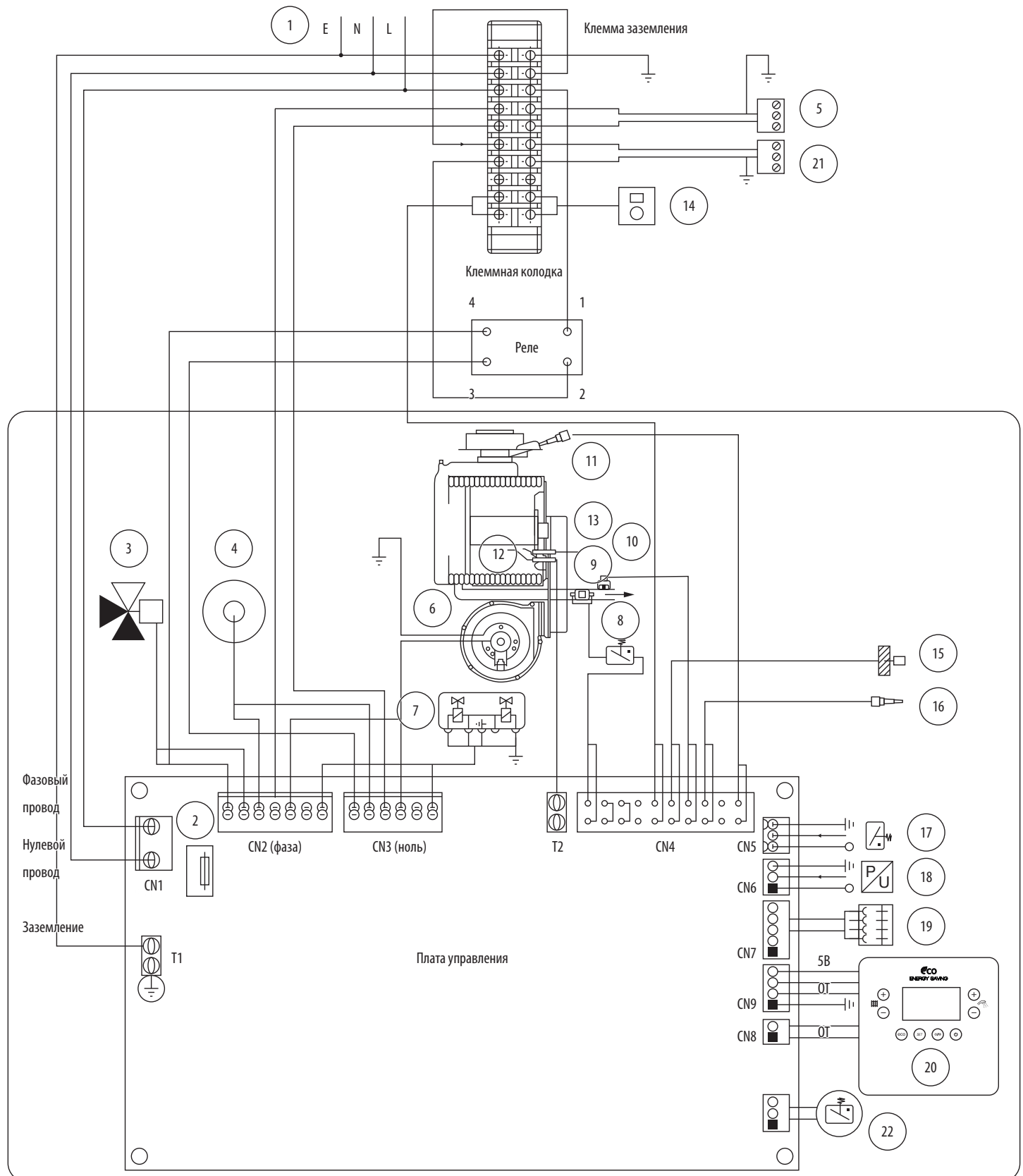
Рис. 41. Электрическая схема платы.
