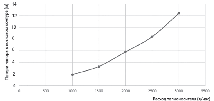
Рис. 42. Потери давления в котловом контуре.
